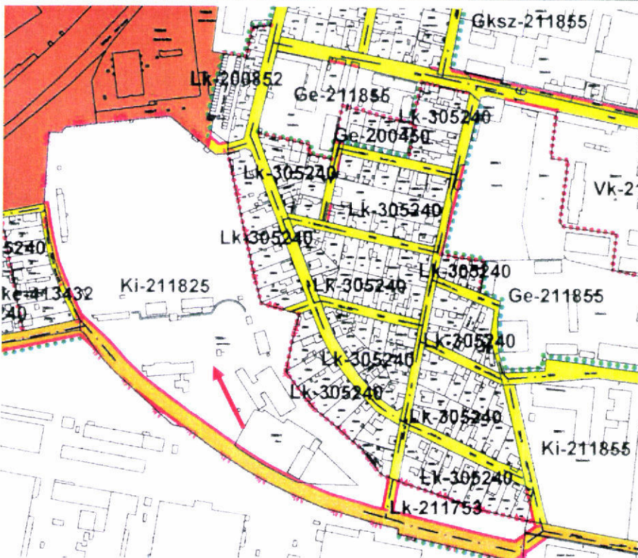
A joghatályos szabályozási tervlap részlete
